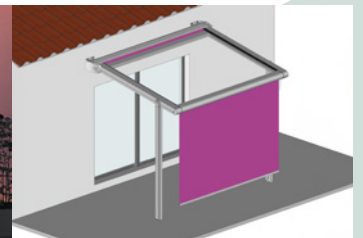
Hauteur du lambrequin : 1500 mm
